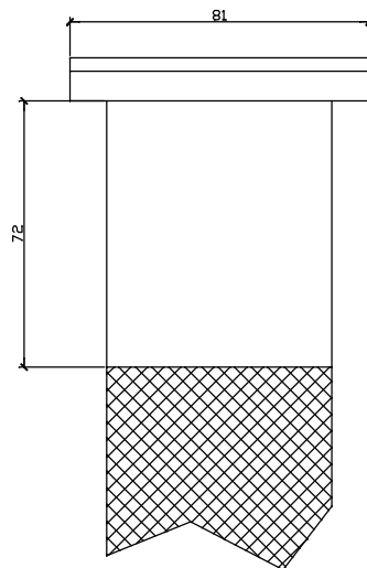
Widok z boku po szerokości kominia
